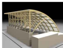
Cubierta para patio de la "Casa de Cultura Bisbe Lorenzana". Girona
